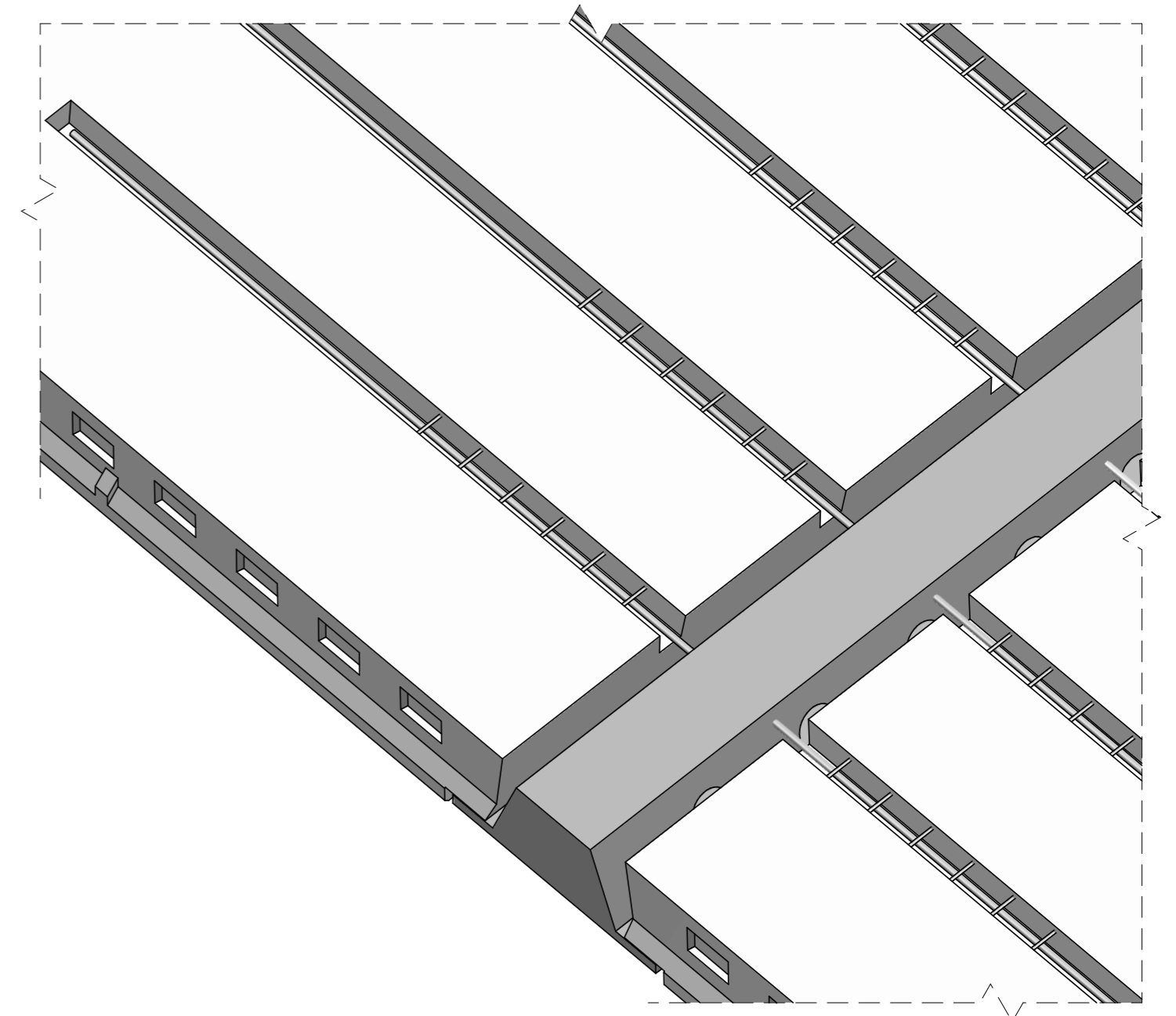
Isometri samling SL-dæk og bjælke (udstøbning ikke vist)
