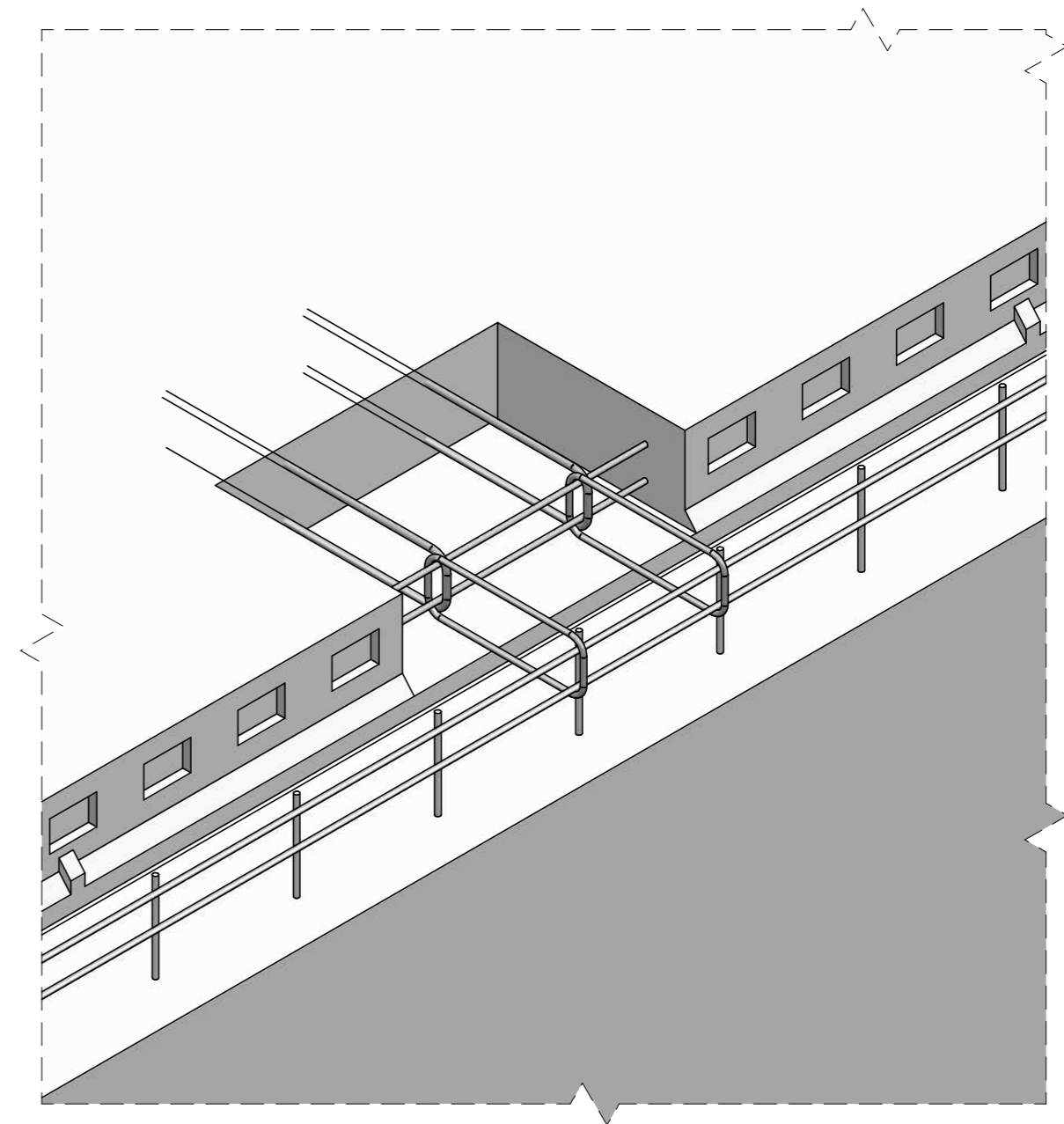
Isometri samling SL-dæk og væg (udstøbning ikke vist)
