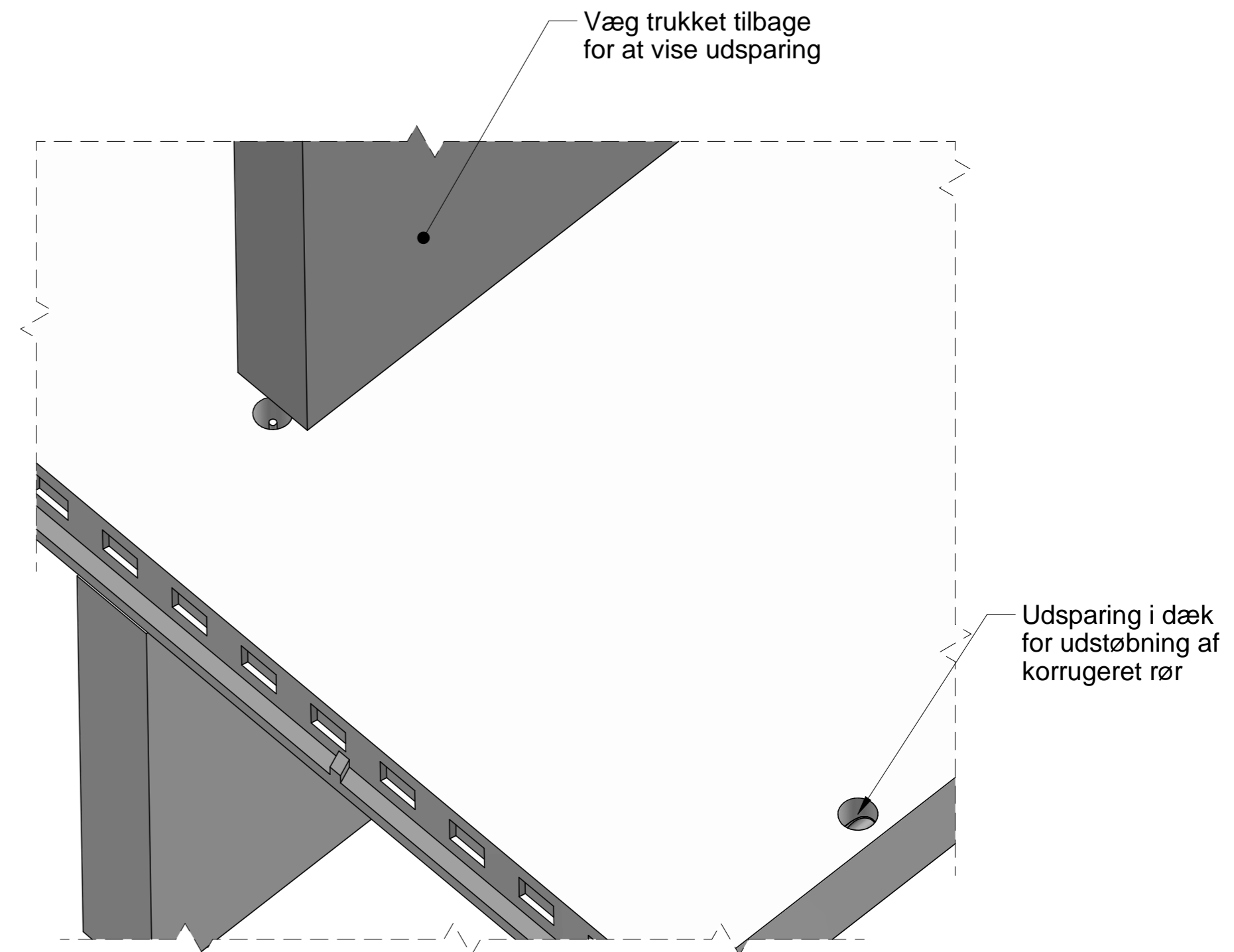
Isometri samling SL-dæk og vægge (udstøbning ikke vist)
